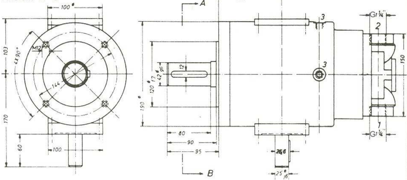
Ansicht A-B
