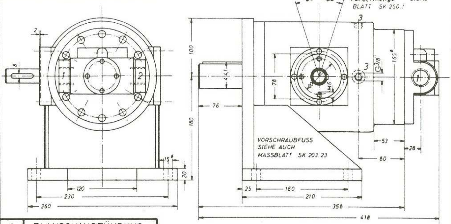
Ansicht A-B
